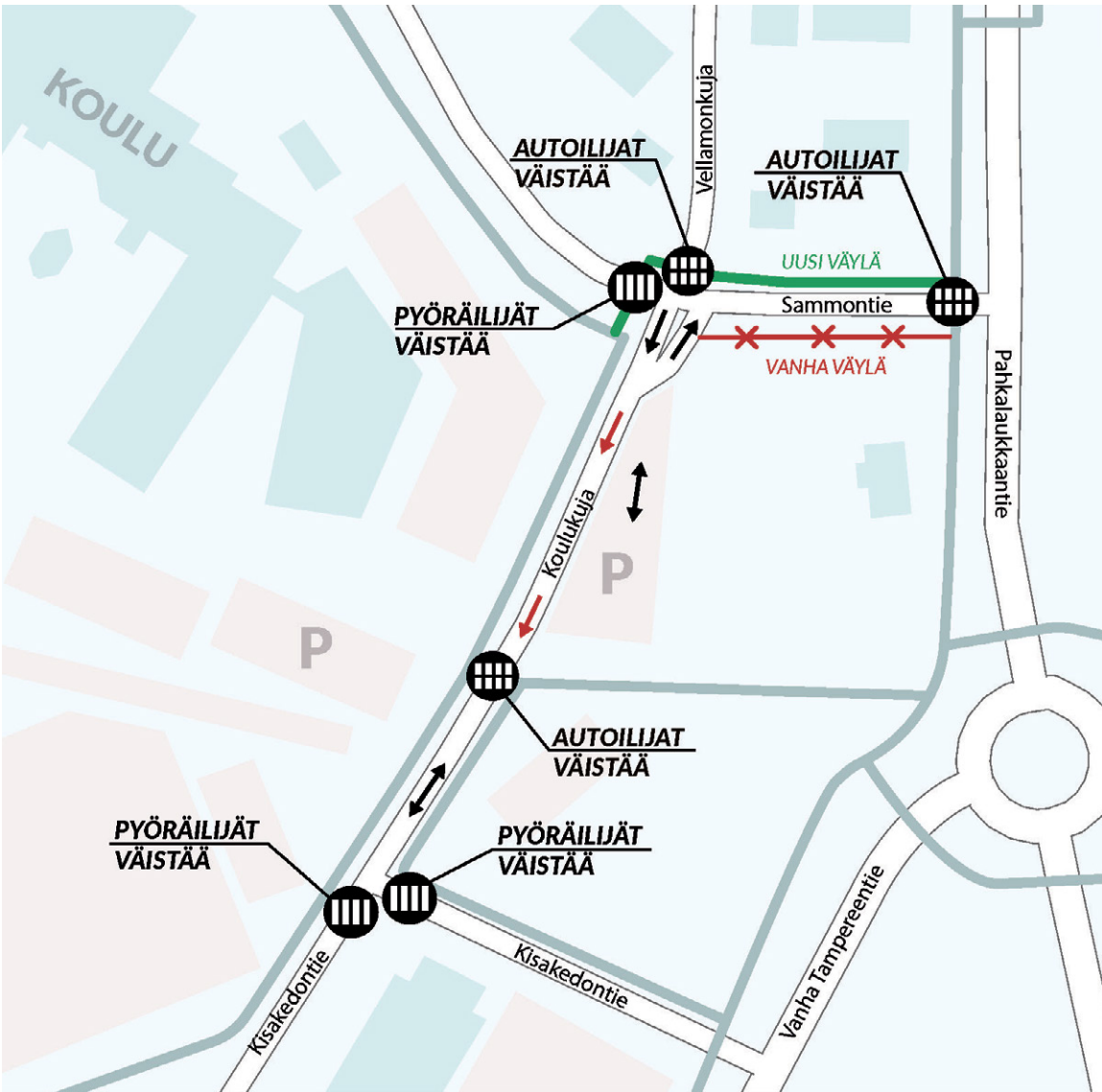
▲ Parannusten yhteydessä muutetaan kevyen liikenteen linjausta, ajo-ohjausta sekä ajosuuntia. Punaisella nuolella on merkitty vain linja-autoille sallittu suunta. Teiden ylityspaikoilla on pyöräilijöiden kannalta eriävät väistämisvelvollisuudet, jotka on tärkeää käydä läpi erityisesti lasten kanssa.
